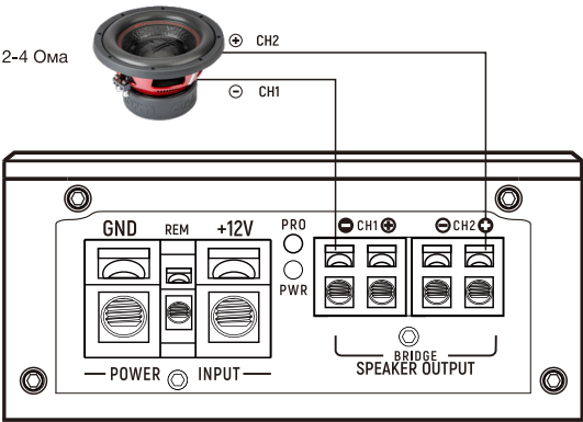
Мостовое подключение
