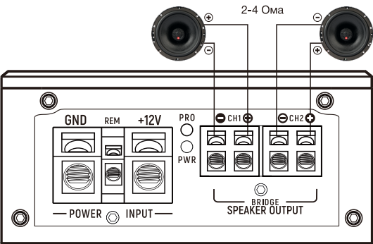
Стерео подключение
