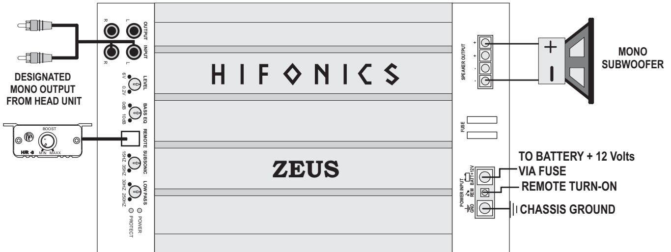
ZRX1200.1D & ZRX1800.1D
