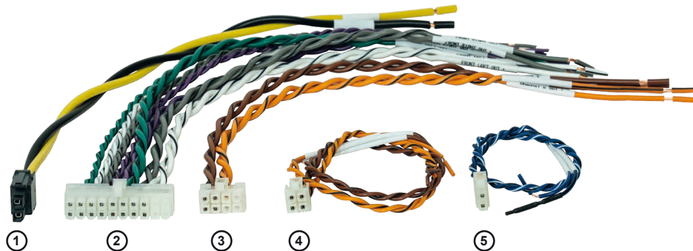
Abb. 2: Übersicht Anschlusskabel
