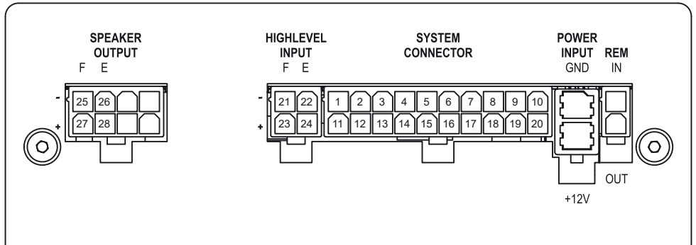
Abb. 1: Pinbelegung UP 6DSP MK2
